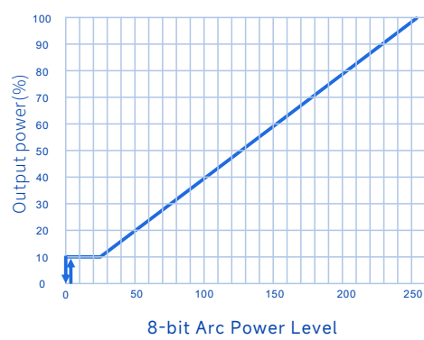
线性调光曲线
